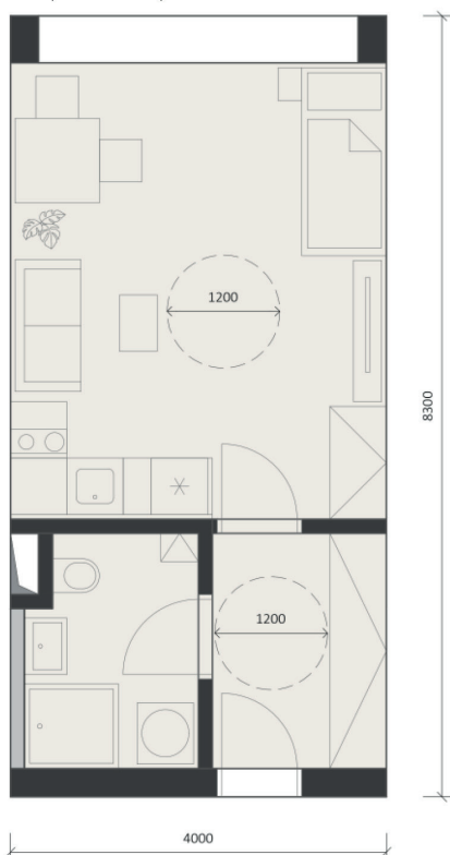
Navržený standardní jednopokojový byt.
